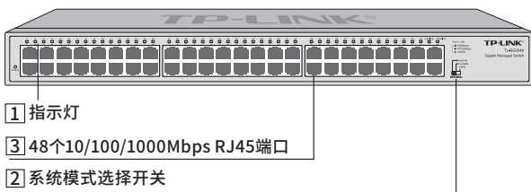
图1-2 TL-SG2048前面板示意图
